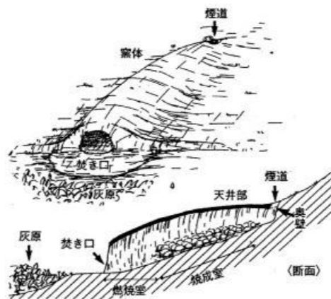
窯構造模式図（山本悦世「寒風古窯跡群」2002から）
