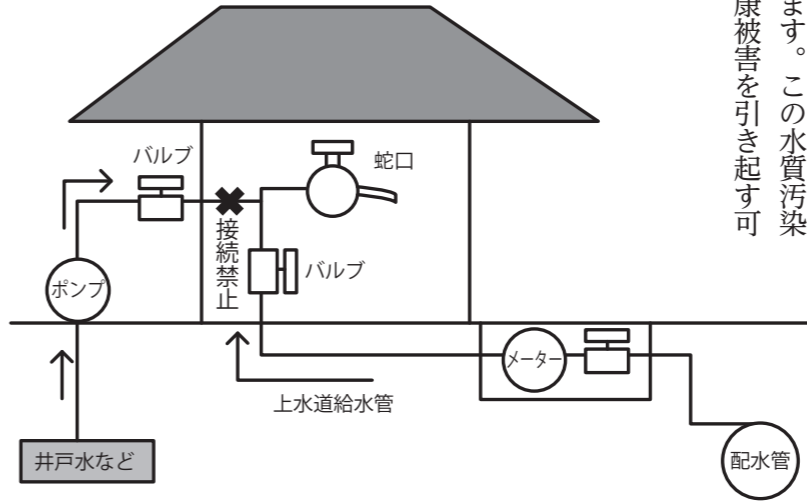
▽給水管への誤接続(クロスコネクション)の例
