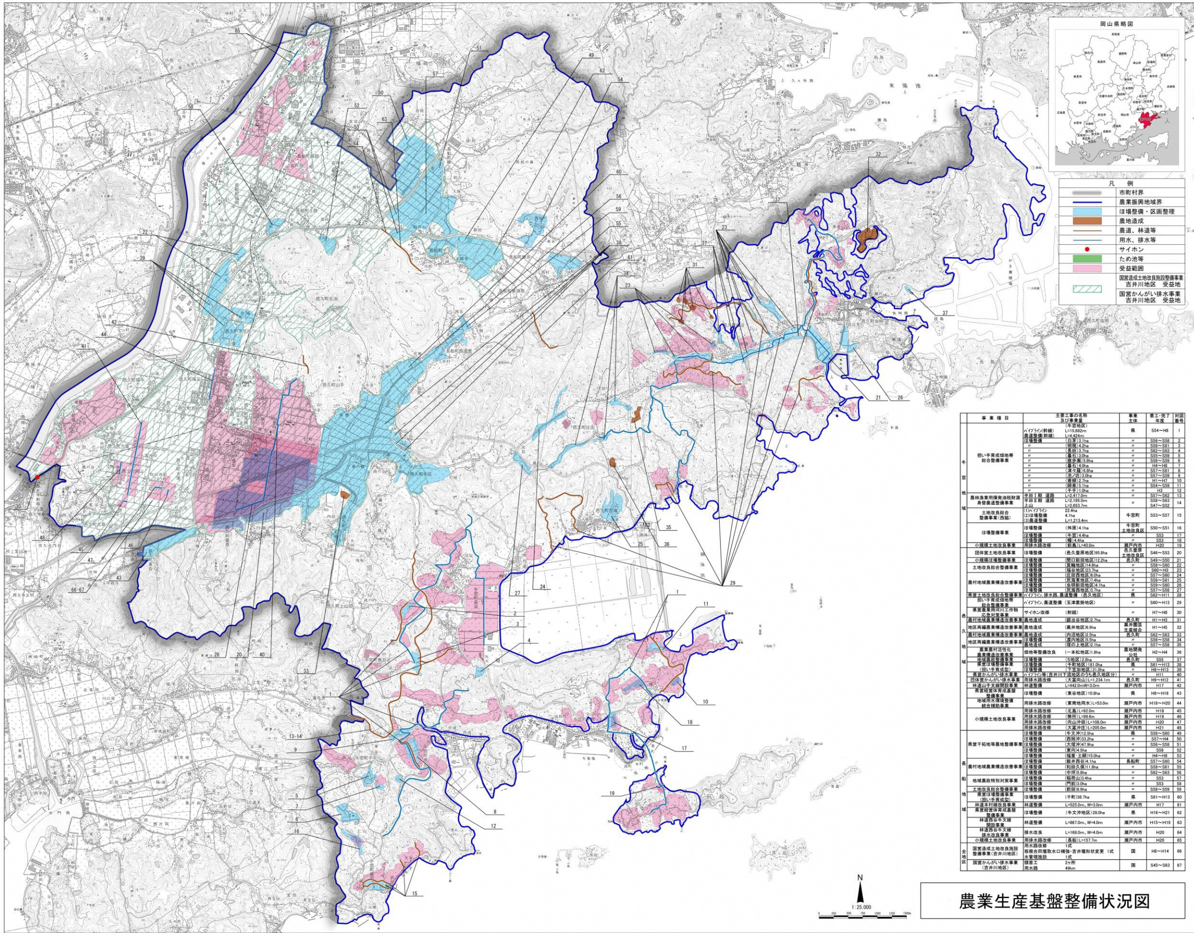
別図-3-① 農業生産基盤の整備開発に係る各種事業の実施状況図(農業生産基盤整備状況図)
