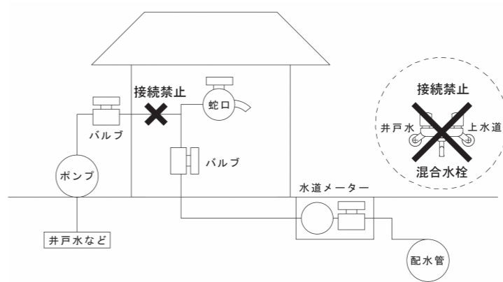
▷クロスコネクションの例
