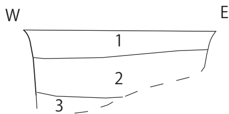
T3 北壁面 (S=1/20)
