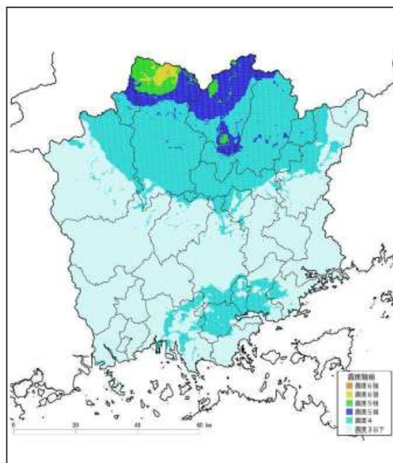
⑥ 大立・田代峠－布江断層
