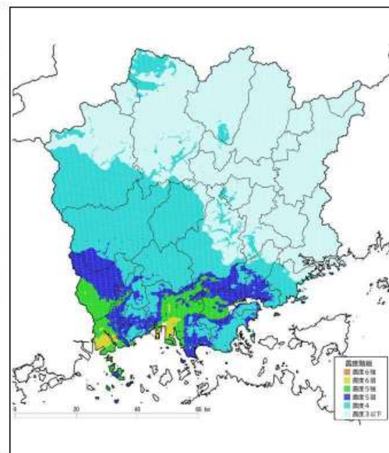
④ 長者ヶ原断層－芳井断層
