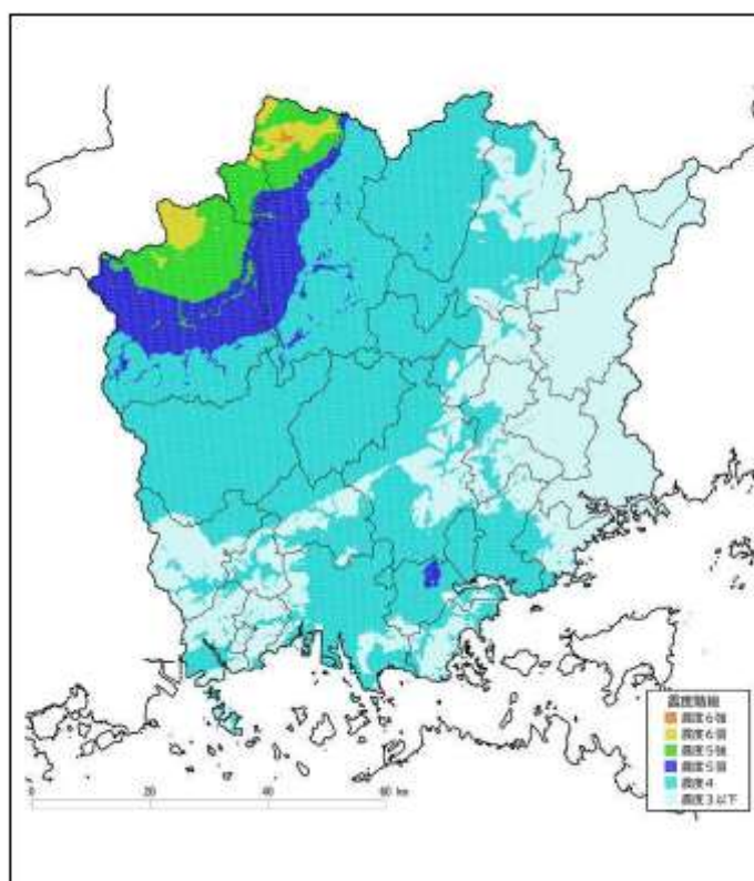
⑦ 鳥取県西部地震
