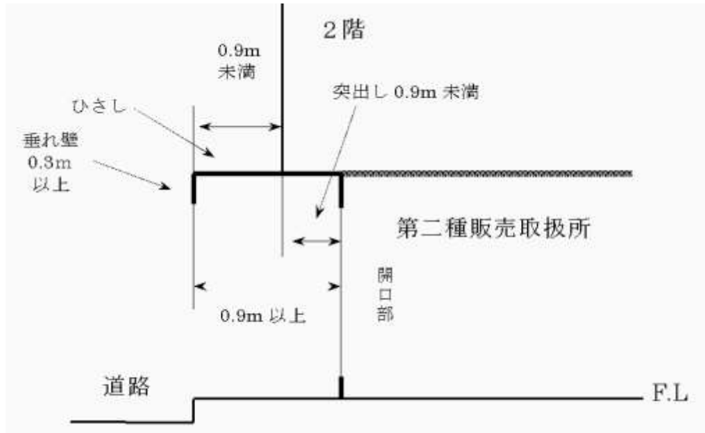
第2-11-6図 側方断面図
