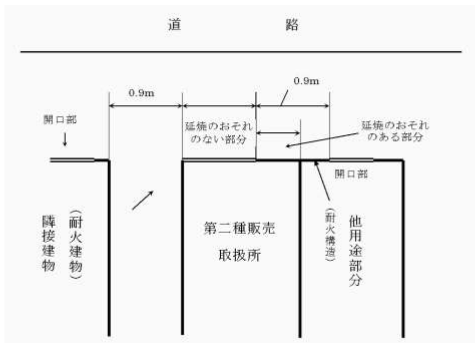
第2-11-7c図 平面図
