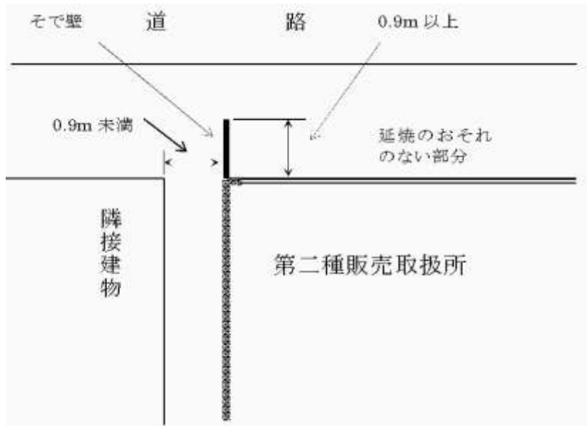
第2-11-8図 平面図
