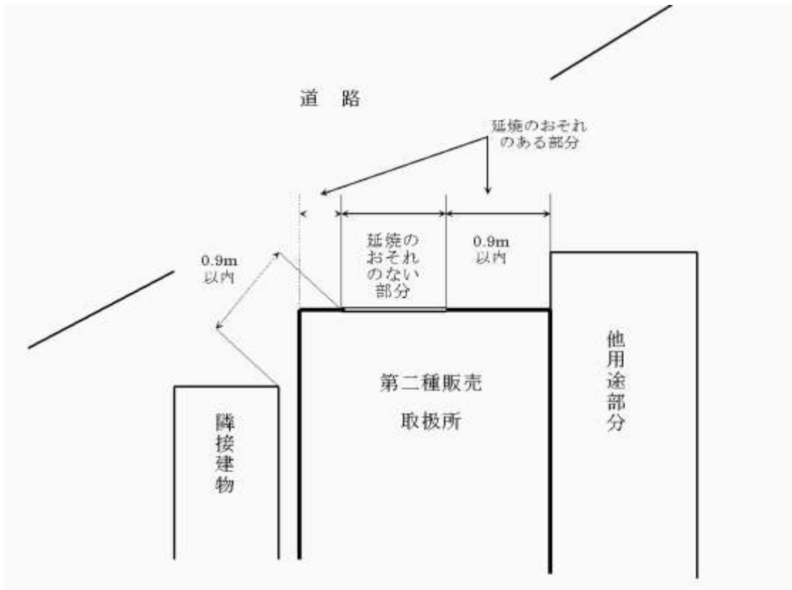
第2-11-7b図 平面図
