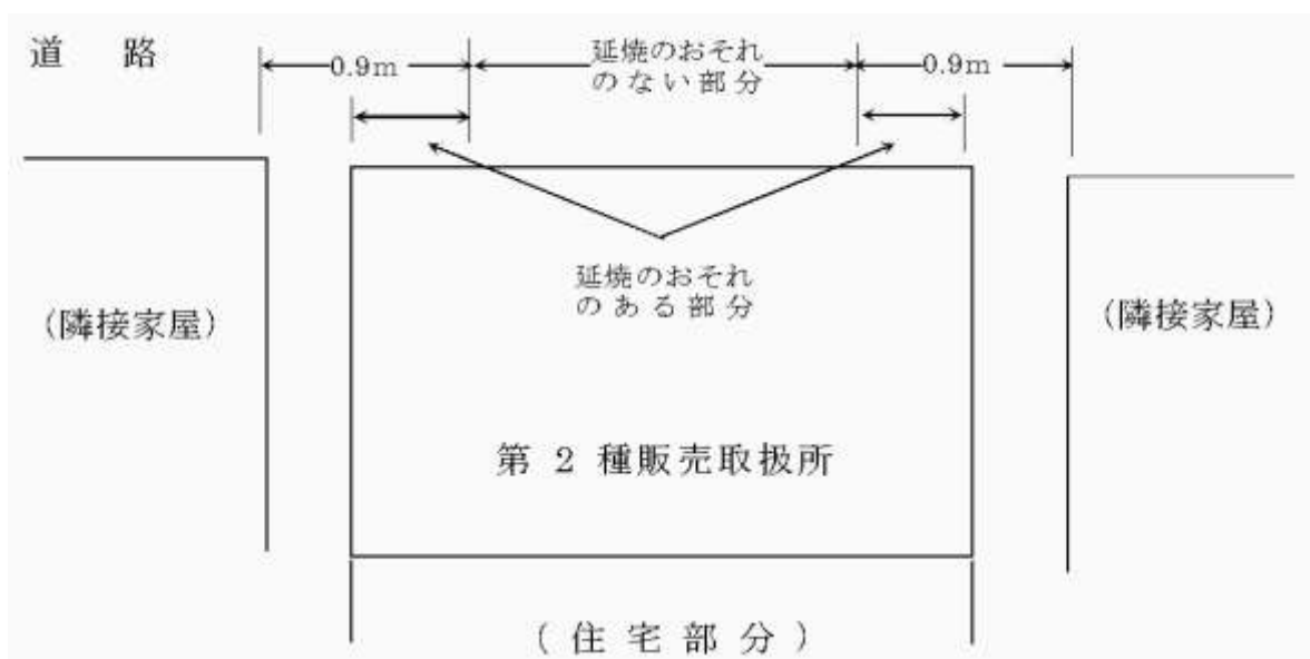
第2-11-7 a 図 平面図
