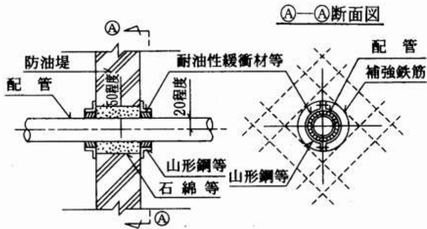
例図2 小口径配管貫通部の保護措置の例
