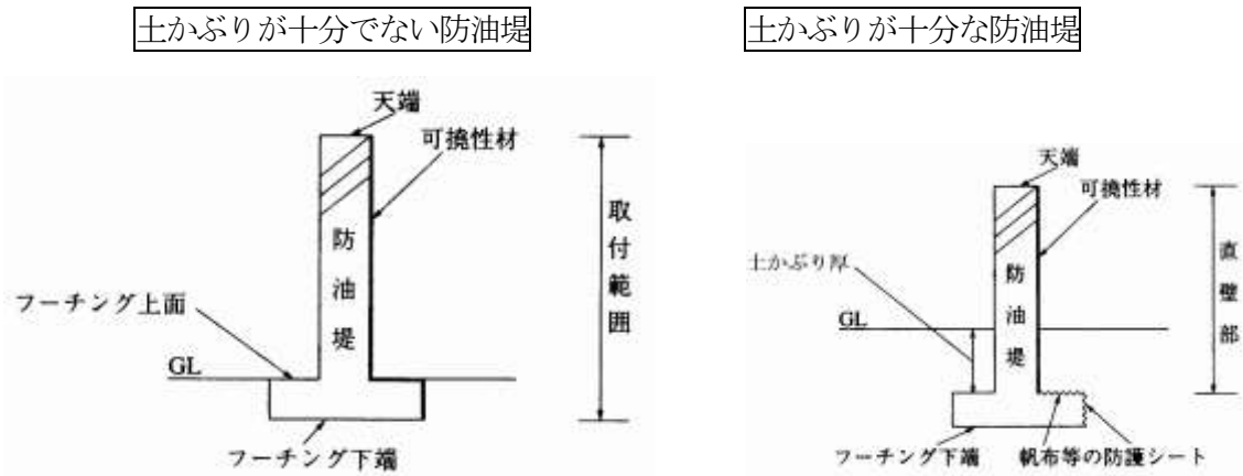
図2 可撓性材の取付範囲
