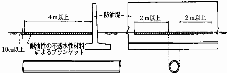
例図6 ブランケットの設置
