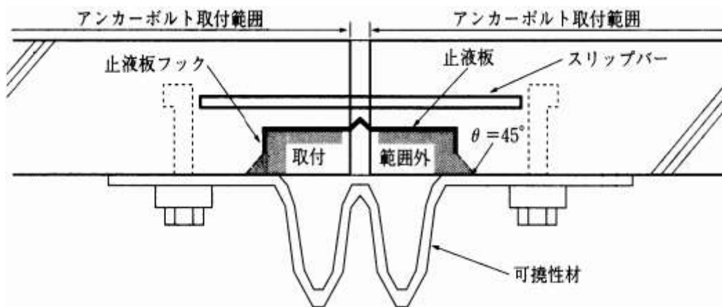
図3 アンカーボルト取付範囲（防油堤目地部を上から見た図）
