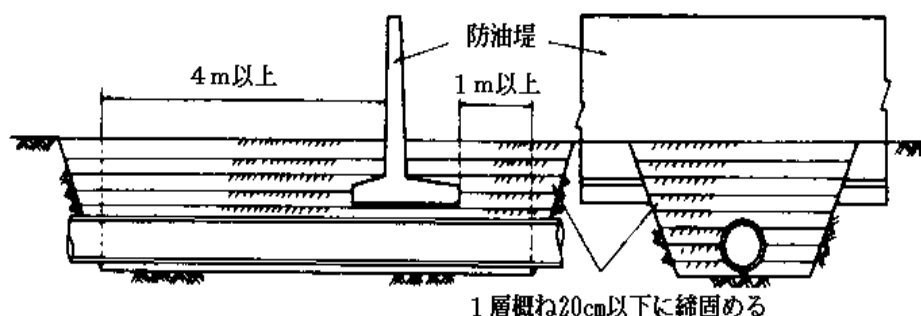
例図4 防油堤築造前に埋設する管渠等の埋戻し要領
